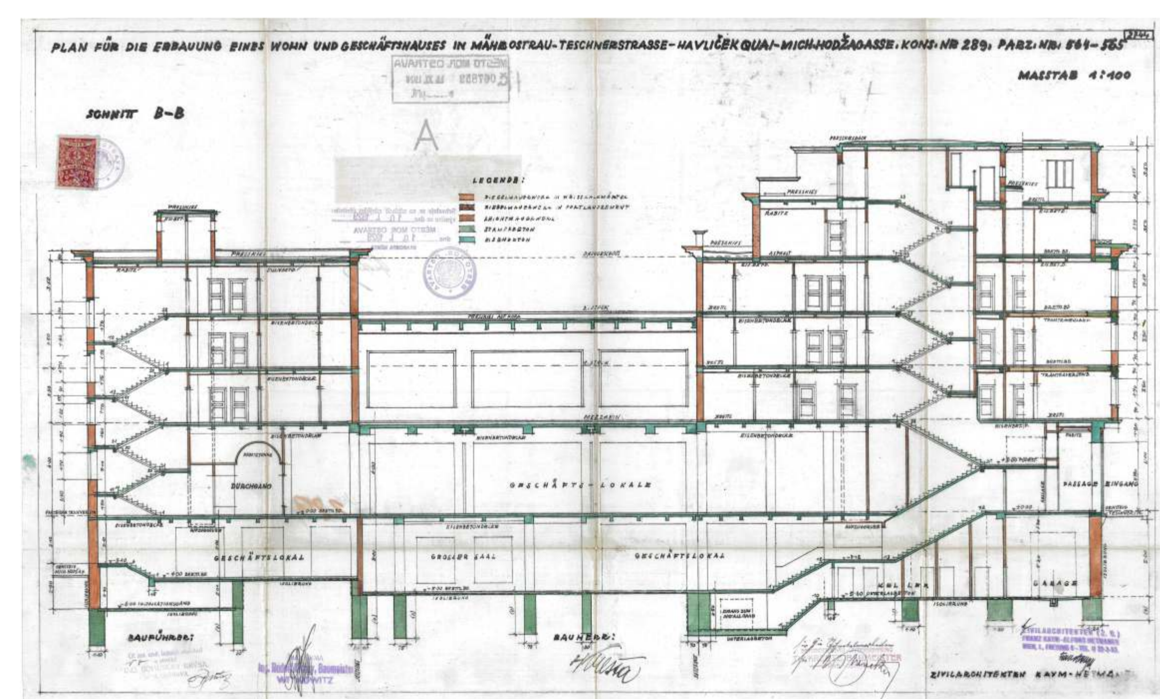
Obr. 5: Obytný a obchodní dům v Moravské Ostravě (1928), společně s Franzem Kaymem, řez z původní projektové dokumentace
